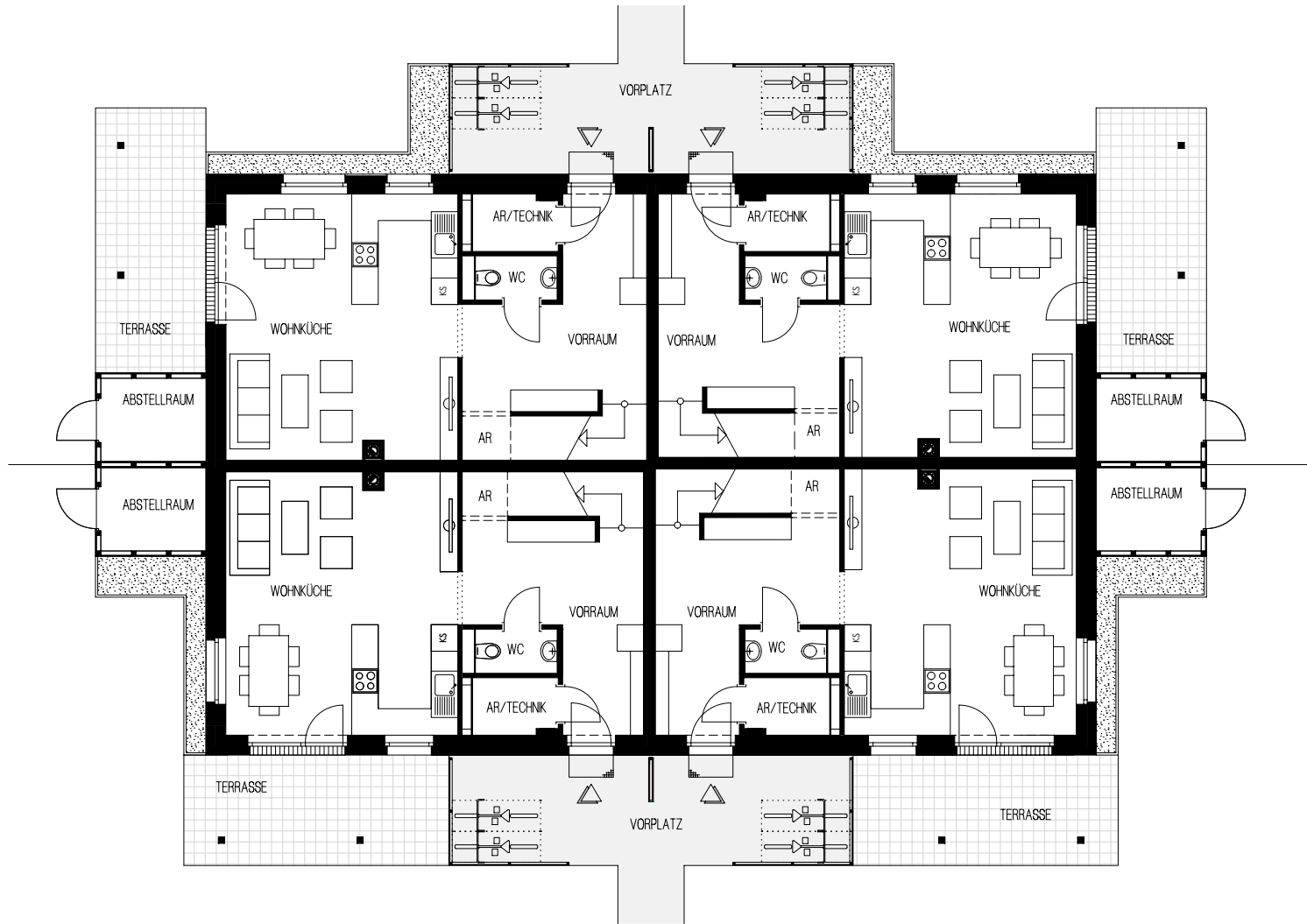
TYP A ERDGESCHOSS AN DER KIPP 21, 23, 25
